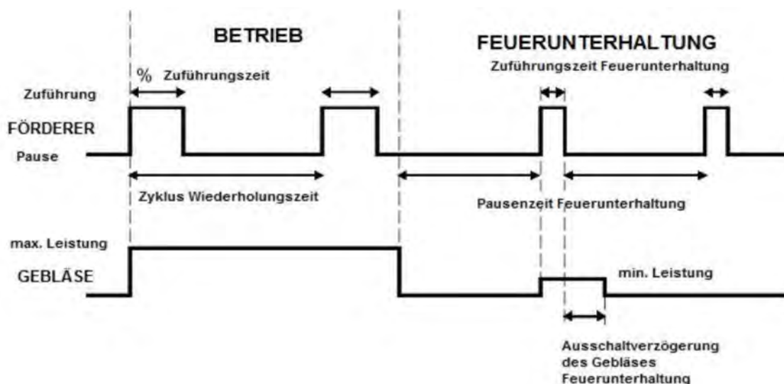
Abbildung 2. Funktionsprinzip des Brennstoff-Förderers und des Gebläses.
