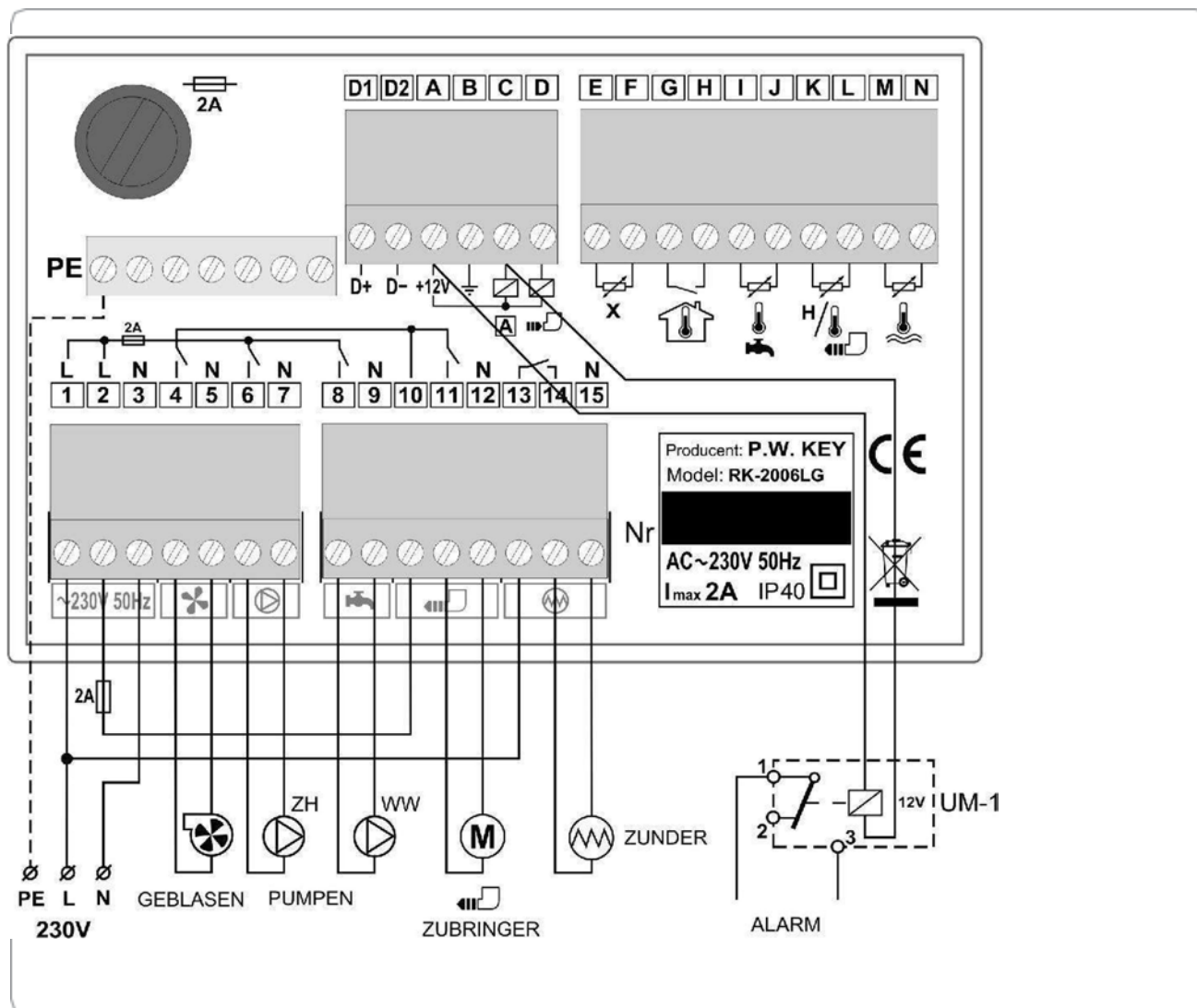
Abbildung 5. Anschlussschema des Reglers RK-2006LG (mit Alarmmeldesystem).
