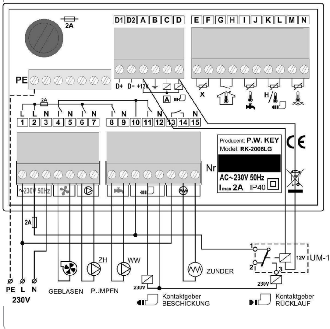
Abbildung 3. Anschlussschema des Reglers RK-2006LG (mit Brennstoff-Rücklaufsystem).
